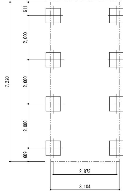
■ 基礎配置図
